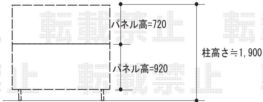
<立面 イメージ図>
