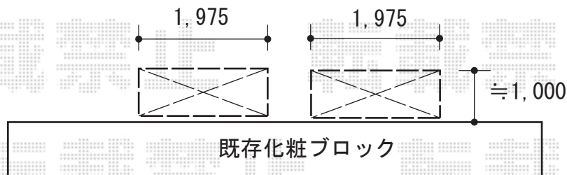
〈正面図〉
