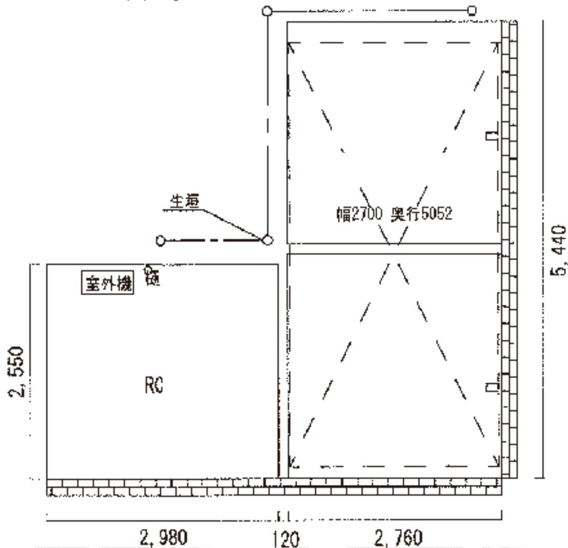
【カーポート 設置図】
