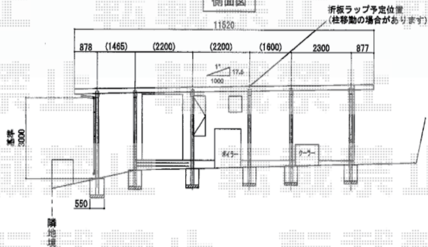
側面図
