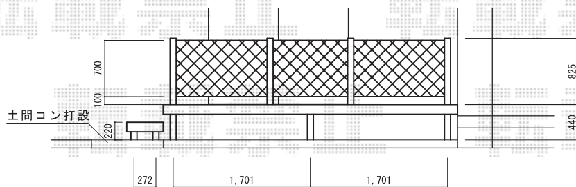
土間コン施工立面図
