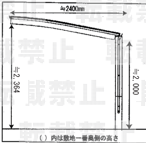
正面図
