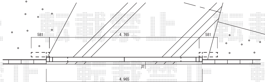
立面図
