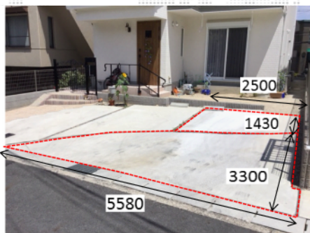
＜土間工事 プラン② 14.2平米＞
