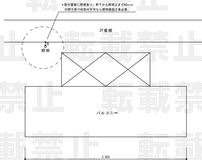
正面図
