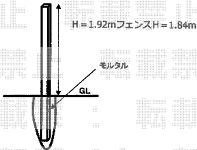
独立多段柱詳細
