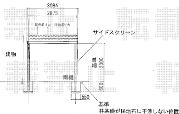
正面図
