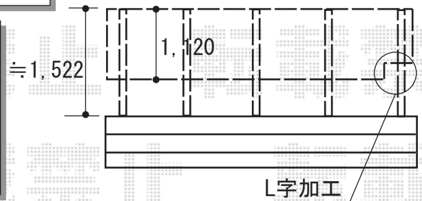
※【01】部分立面図
