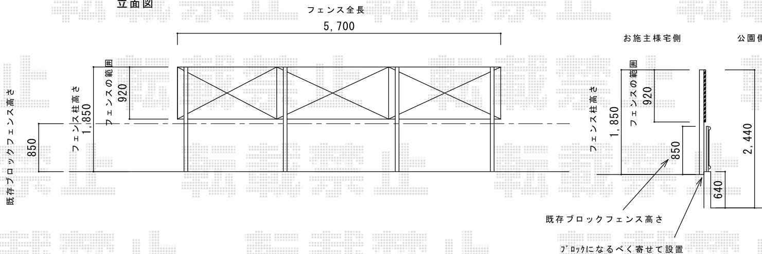
立面図
