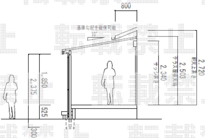
側面図 1/80
