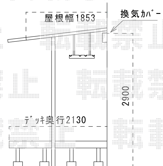
側面図
