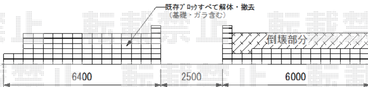
現況側面図
