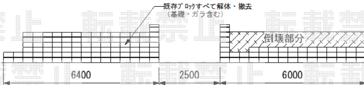
現況側面図
