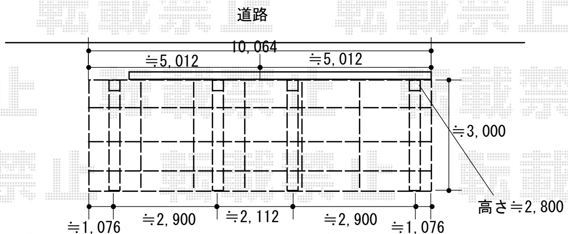
平面図
