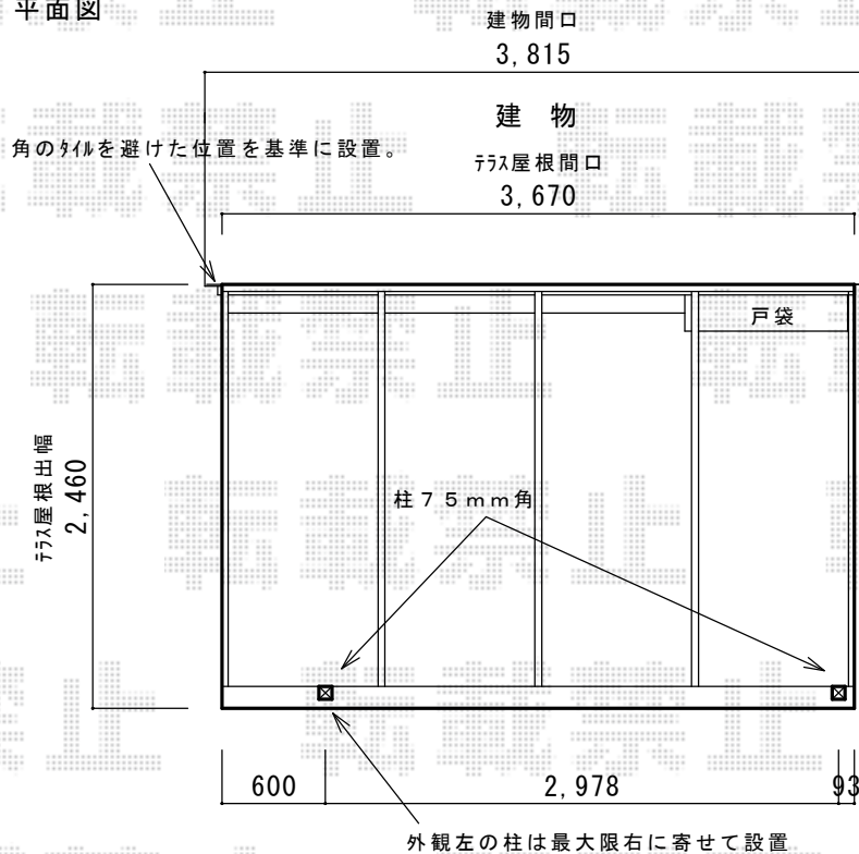
平面図
