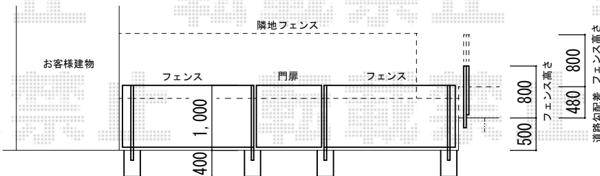
庭側立面図
