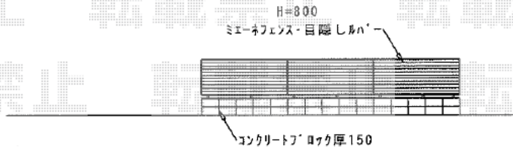
[A] 計画立面図
