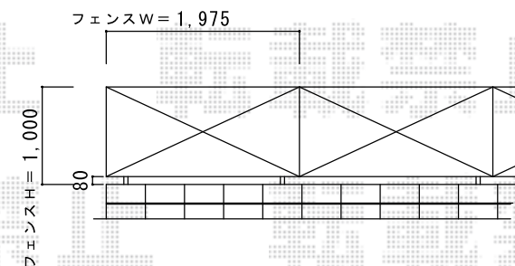
立面図
