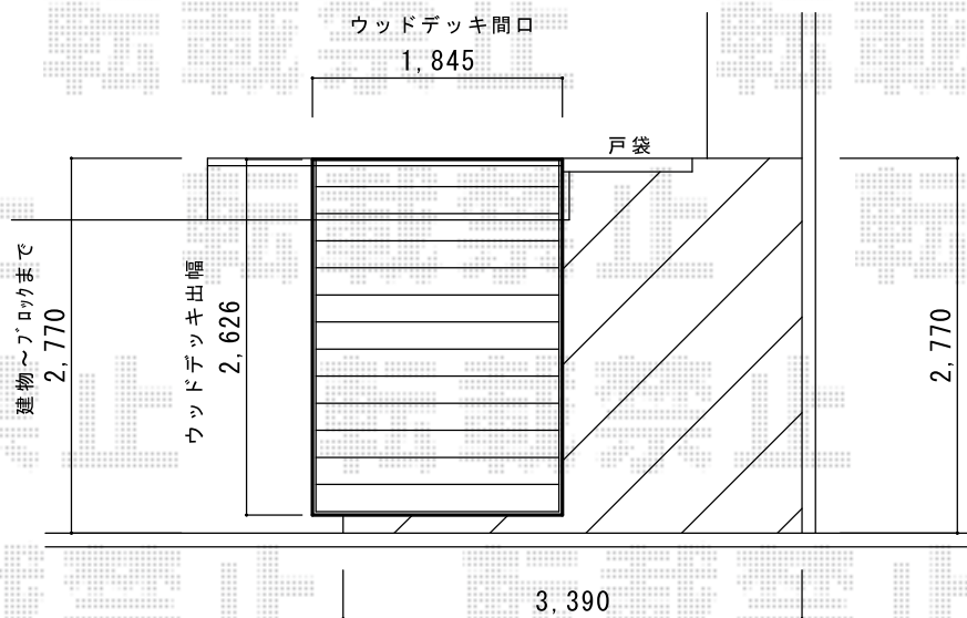
平面図
