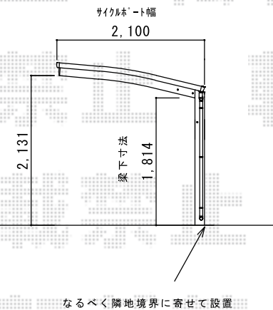
立面図
