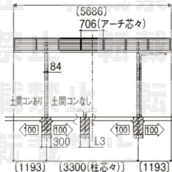
●基本(雨樋有り):側面図
