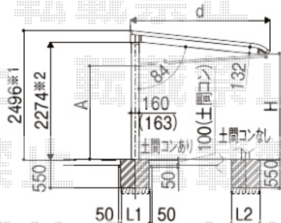
●基本・延長・縦連棟(雨樋有り):正面図
