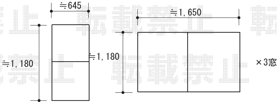
面格子
