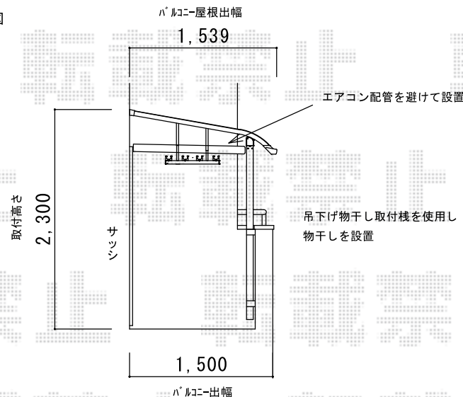
立面図
