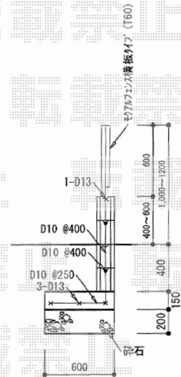
断面図
