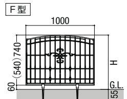
柱外形寸法(G.L部)=25×17 ( )T-6の場合
