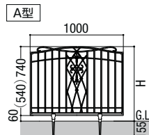
柱外形寸法(G.L部)=25×17 ( )T-6の場合
