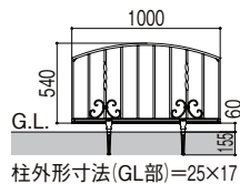
柱外形寸法(G.L部)=25×17
