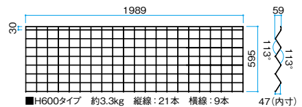
■H600タイプ 約3.3kg 縦線：21本 横線：9本 ※高さ595は最上部と最下部の横線の芯々寸法
