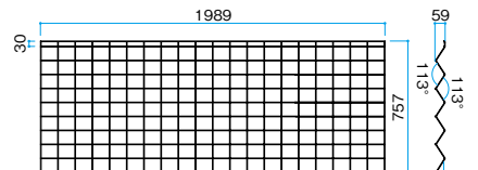
■H800タイプ 約4.2kg 縦線：21本 横線：11本 ※高さ757は最上部と最下部の横線の芯々寸法
