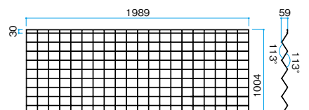
■H1000タイプ 約5.5kg 縦線：21本 横線：14本 ※高さ1004は最上部と最下部の横線の芯々寸法
