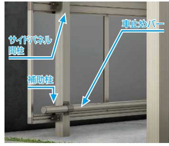
補助柱付き車止めバー プラチナステン色
